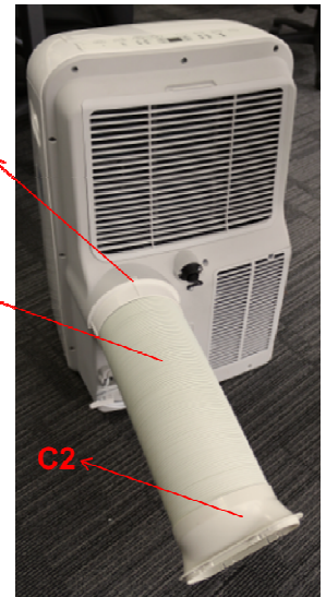
Použitie nástavca na vyplnenie otvoru okna
