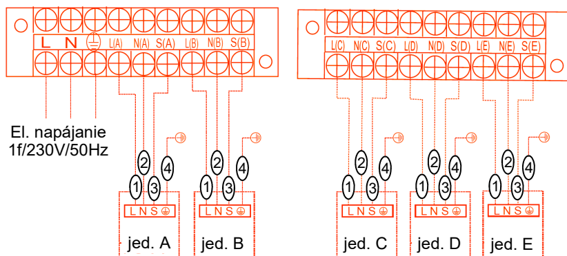
Svorkovnice YDZC 5-42:
