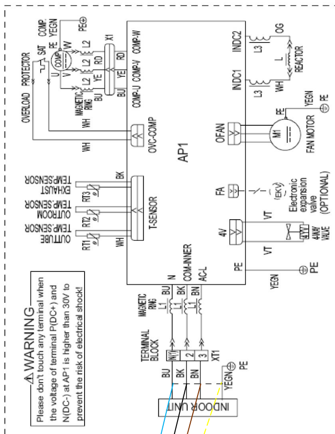
Vonkajšia jednotka GC YDDE 018 DCI
