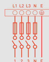
Třífázové napájení 3 x 400 V / 1 N – 50 Hz / *
