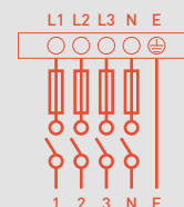
Třífázové napájení 3 x 400 V / 1 N – 50 Hz / **
