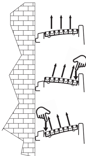
2.14 Luftzufuhrgitter - Ausrichtung des Luftstroms - nur YFTS-ECM-VC
