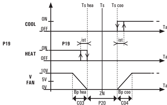
Fig. 11: Lo schema mostra il pilotaggio delle valvole in un impianto a 4 tubi con zona neutra. Analogamente, l'uscita valvola caldo ( HEAT ) di un sistema a 2 tubi verrà pilotata allo stesso modo, in questo caso la T_s (temperatura di setpoint) coinciderà con T_s \text{ ris} in inverno e T_s \text{ raf} in estate.
