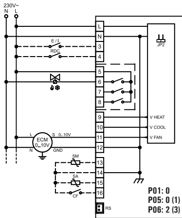
Fig. 9: Schema di collegamento per pilotaggio di un attuttore on/off a 230V ~ per impianto a 2 tubi e pilotaggio proporzionale del ventilatore. Wiring diagram for 1 on/off 230V ~ actuators in 2 pipes system and proportional fan drive.
