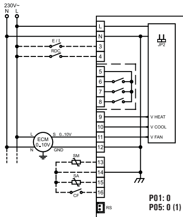
Fig. 10: Schema di collegamento per pilotaggio proporzionale del ventilatore.
