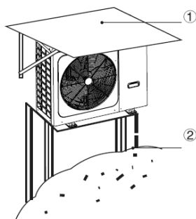
1 - strieška proti snehu 2 - konzola, podstava
