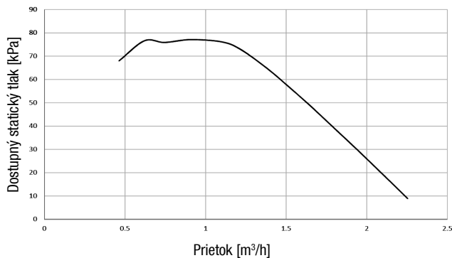
Dostupný statický tlak ESP vs. prietok
