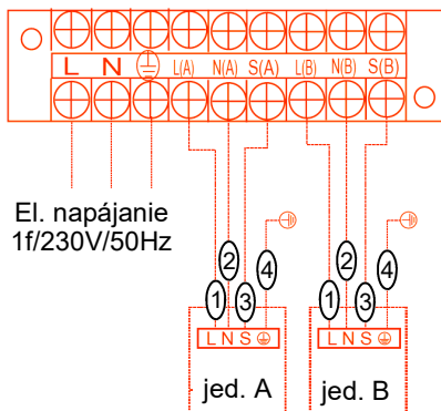
Svorkovnice YDZC 5-42:
