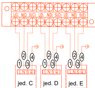
Svorkovnica HKD 2019:
