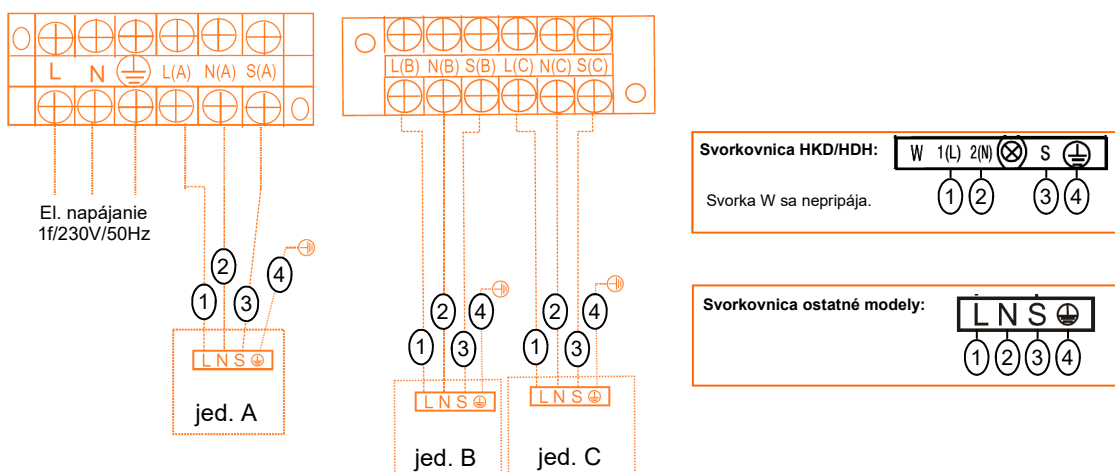
Svorkovnice YDZC 3-27:
