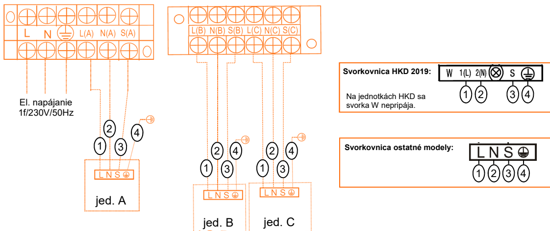
Svorkovnice YDZC 3-27:
