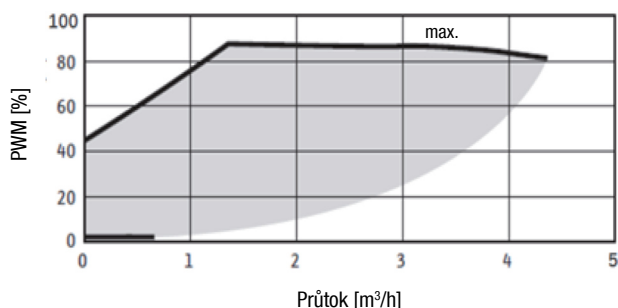
Závislost mezi PWM a průtokem:
