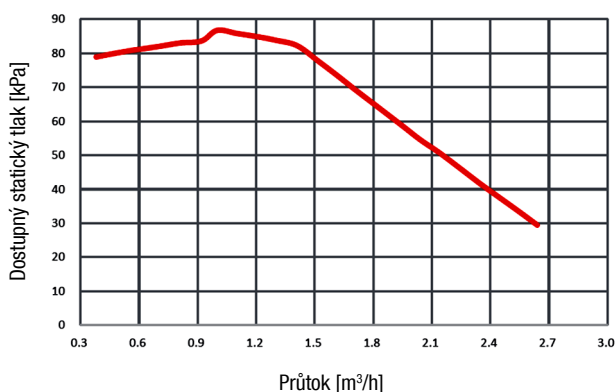
Dostupný statický tlak ESP vs. průtok (modely 4-10kW):
