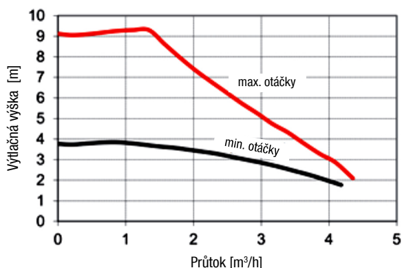
Závislost mezi výtlačnou výškou a průtokem (regulační rozsah je mezi křivkou min. a max. otáček):
