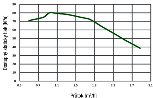
Dostupný statický tlak ESP vs. průtok (modely 12-16kW):
