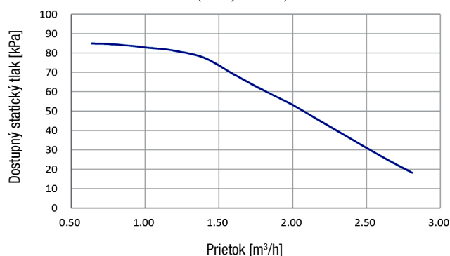
Dostupný statický tlak ESP vs. prietok (modely 12-16kW):
