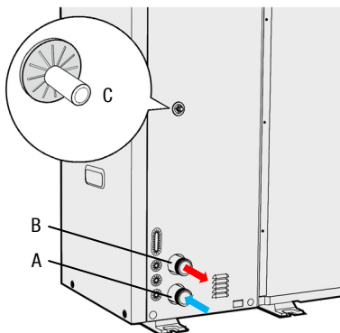
A - vstup vody (water inlet) 1 1/4", B - výstup vody (water outlet) 1 1/4", C - odtok z poistného ventilu
