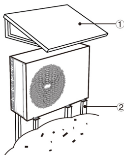
1 - strieška proti snehu 2 - konzola, podstava
