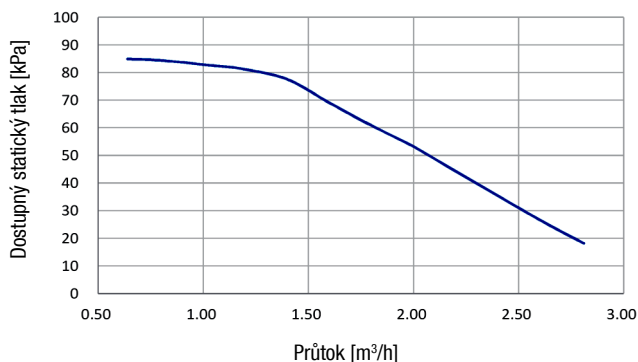
Dostupný statický tlak ESP vs. průtok (modely 12-16kW):
