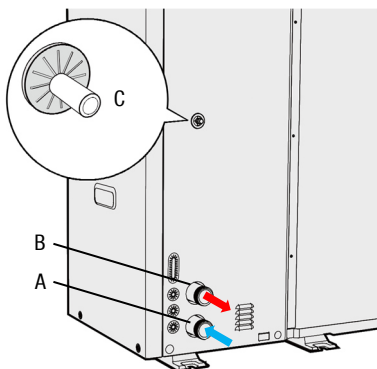
A - vstup vody (water inlet) 1 1/4", B - výstup vody (water outlet) 1 1/4", C - odtok z pojistného ventilu
