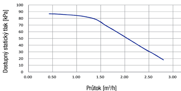
Dostupný statický tlak ESP vs. průtok (modely 12-16kW):
