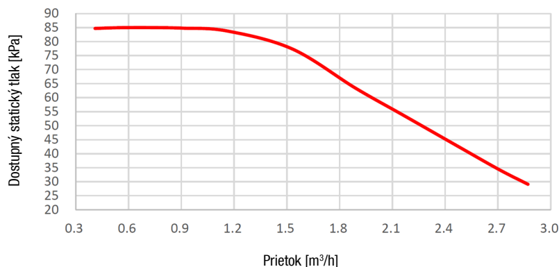
Dostupný statický tlak ESP vs. prietok
