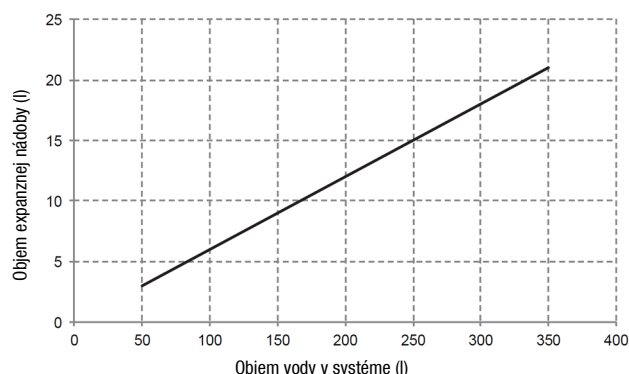
Objem expanznej nádoby vs. objem vody v systéme:
