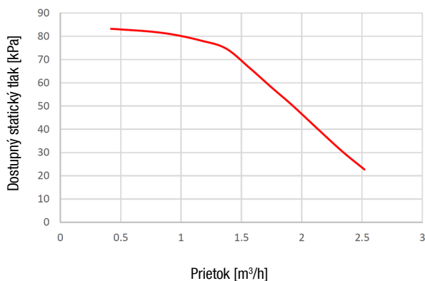
Dostupný statický tlak ESP vs. prietok
