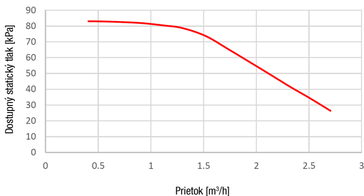
Dostupný statický tlak ESP vs. prietok
