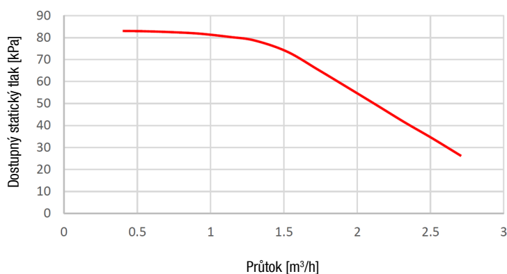
Dostupný statický tlak ESP vs. průtok
