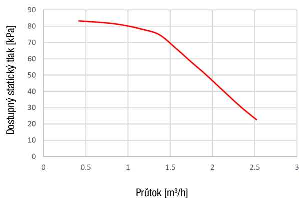
Dostupný statický tlak ESP vs. průtok
