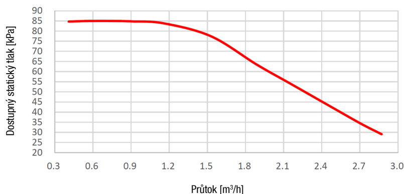
Dostupný statický tlak ESP vs. průtok
