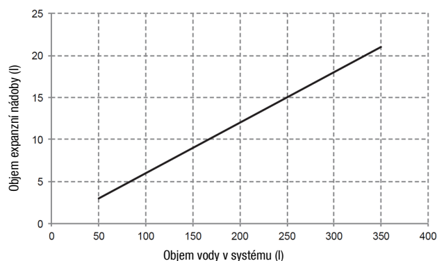
Objem expanzní nádoby vs. objem vody v systému:
