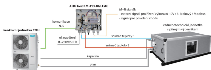
Schéma přepojení LCAC:
