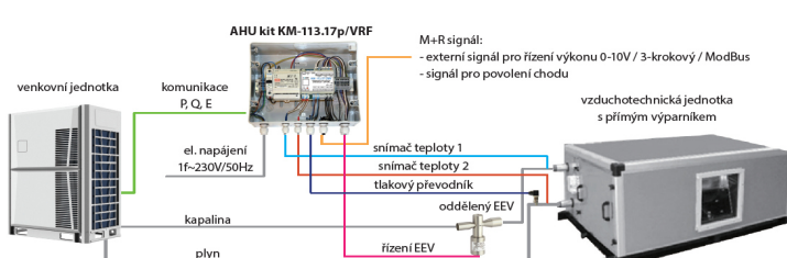
Schéma přepojení VRF:
